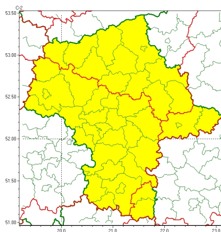
Silny wiatr 2023-11-22 12:12
